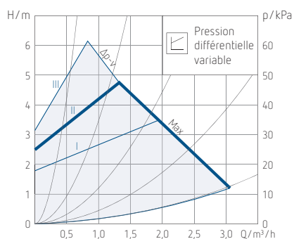
Réglage préférentiel pour une installation avec radiateurs ou plancher chauffant. La vitesse du circulateur s'adapte pour faire varier la pression.
