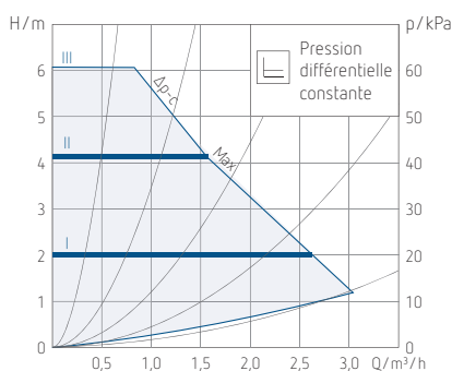
Réglage préférentiel pour une installation en plancher chauffant. La vitesse du circulateur s'adapte pour maintenir la pression constante.
