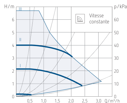
Réglage préférentiel pour un circuit dont les pertes de charge ne varient pas. La vitesse du circulateur est constante.
